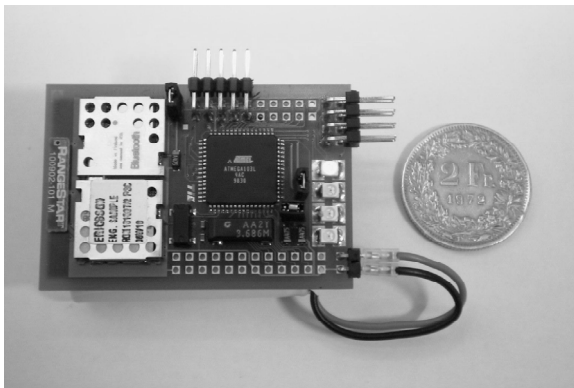
Ein im Rahmen des „Disappearing Computer“-Programms entwickeltes „Smart-It“: Angeheftet an Gegenstände sendet es Sensorinformation via Bluetooth an andere Gegenstände (ETH Zürich).
